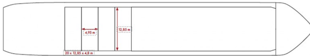
Tween Deck
